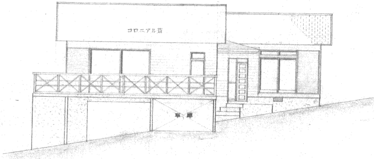
南面立 面 図 S = 1/100
