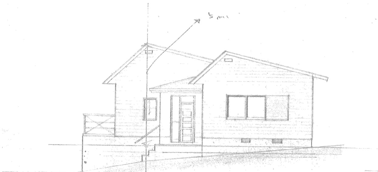
東面立面 図 S = 1/100
