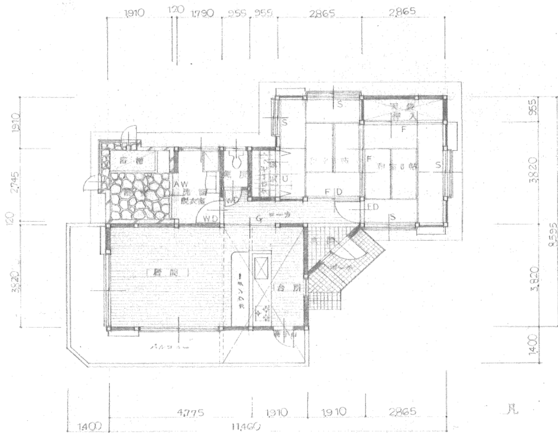
階平面図 S = 1/100
